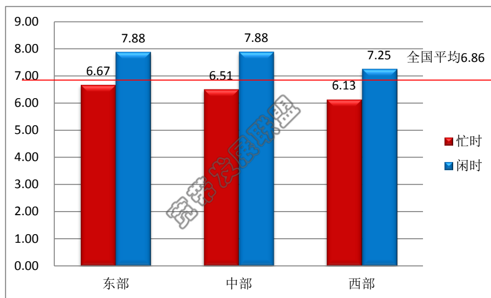
图15 忙、闲时平均视频下载速率区域对比（单位：Mbit/s）
