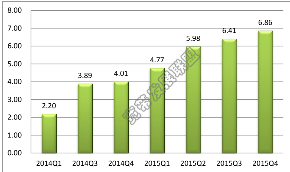
图13 2014年第一季度至本季度全国平均视频下载速率对比（单位：Mbit/s）
