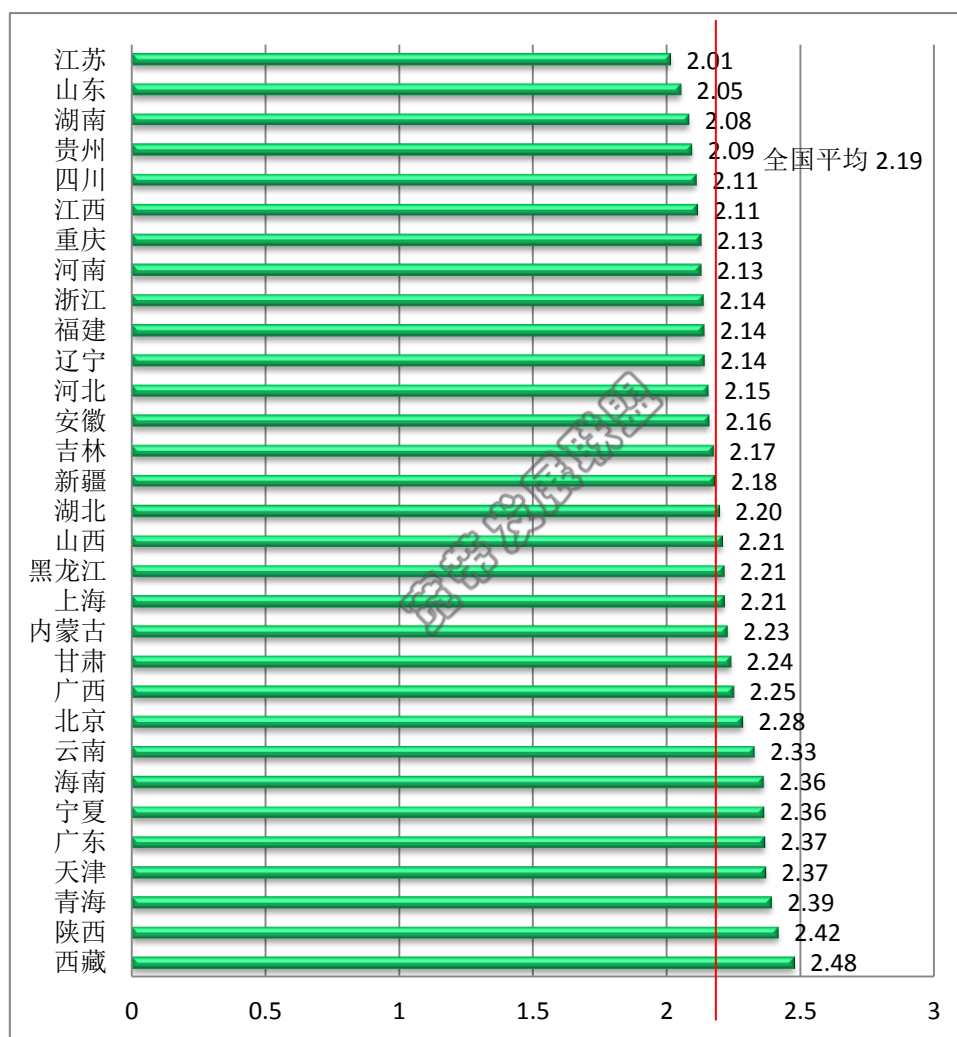
图11 各省忙闲时加权平均首屏呈现时间 (单位: s)
